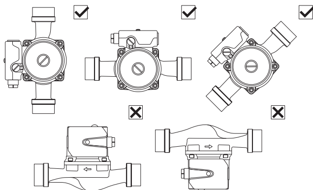
Рис. 7. Варианты расположения насоса
