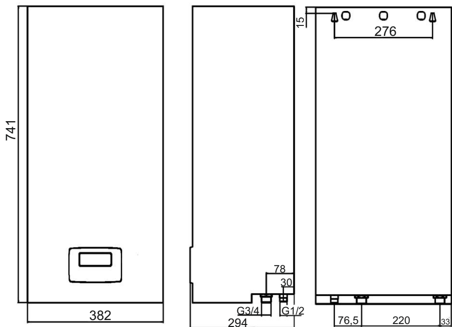
Рисунок 12. Габаритные и присоединительные размеры прибора
