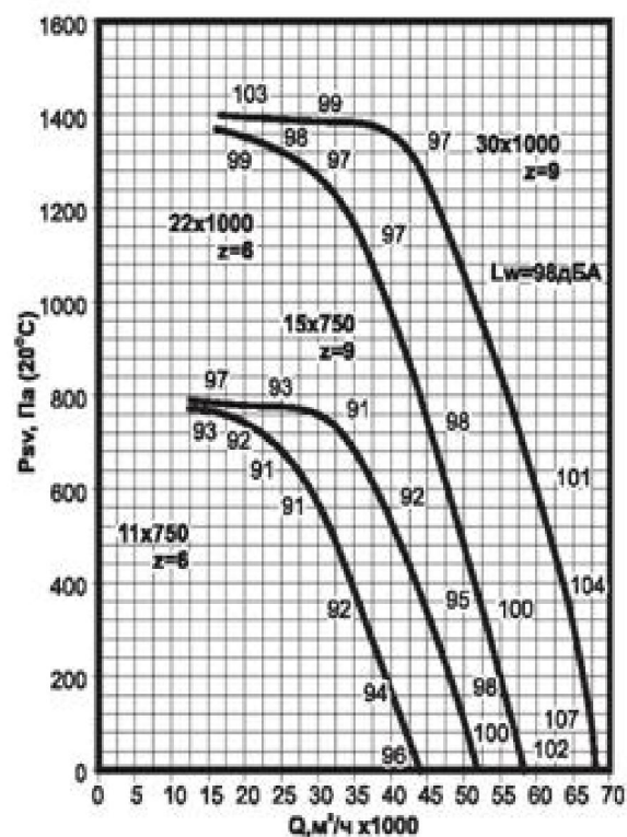
Аэродинамическая характеристика ВКРФ №11,2
