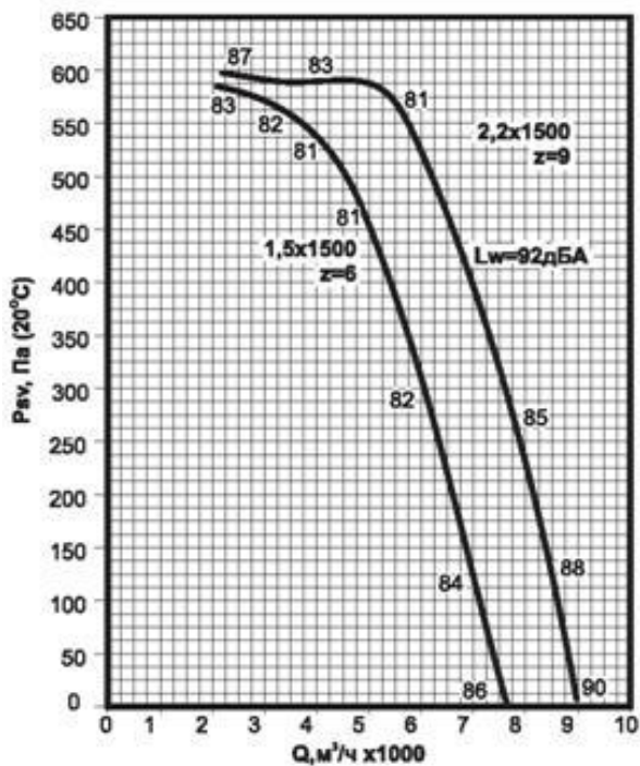
Аэродинамическая характеристика ВКРФ №5
