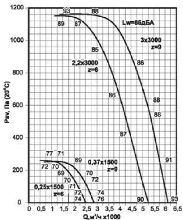
Аэродинамическая характеристика ВКРФ №3,55
