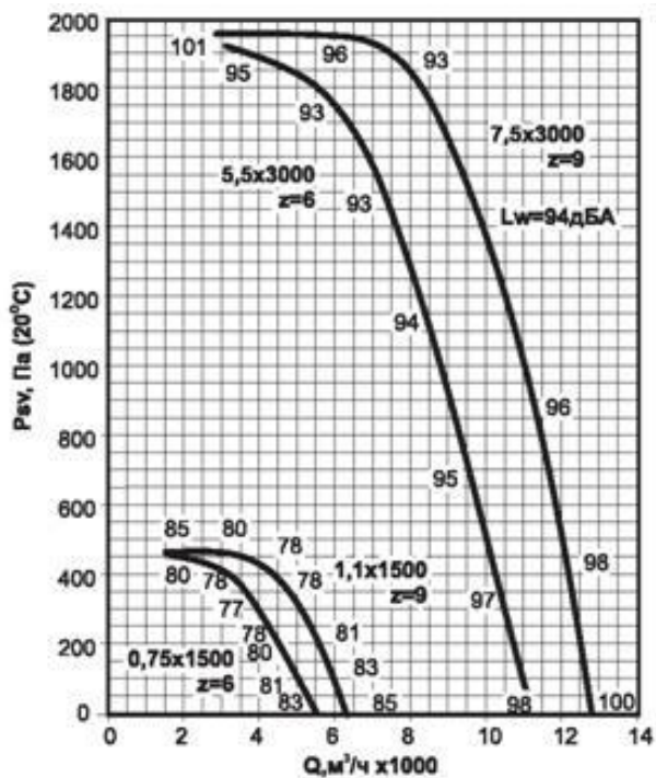
Аэродинамическая характеристика ВКРФ №4,5
