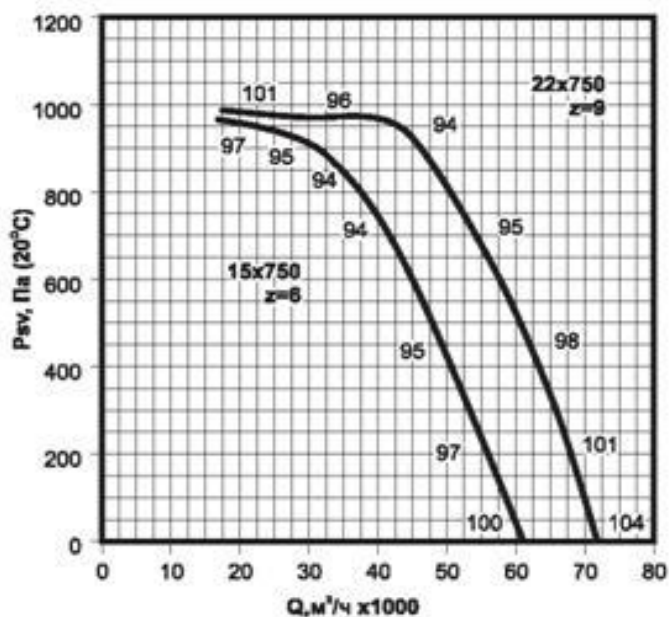
Аэродинамическая характеристика ВКРФ №12,5
