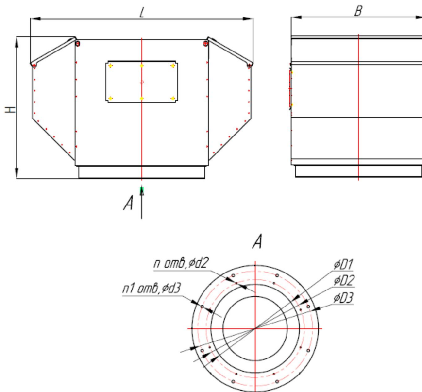
Габаритные и присоединительные размеры вентиляторов крышных типа ВКРФ 3,55-12,5
