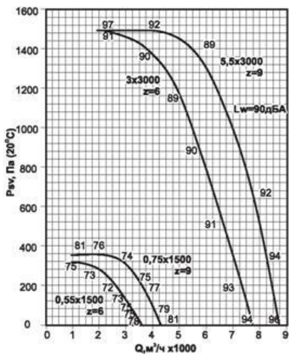
Аэродинамическая характеристика ВКРФ №4
