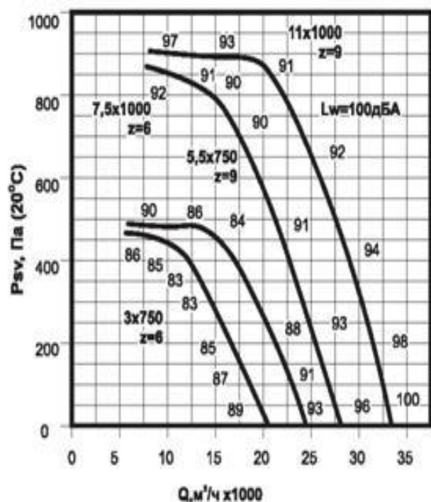
Аэродинамическая характеристика ВКРФ №9
