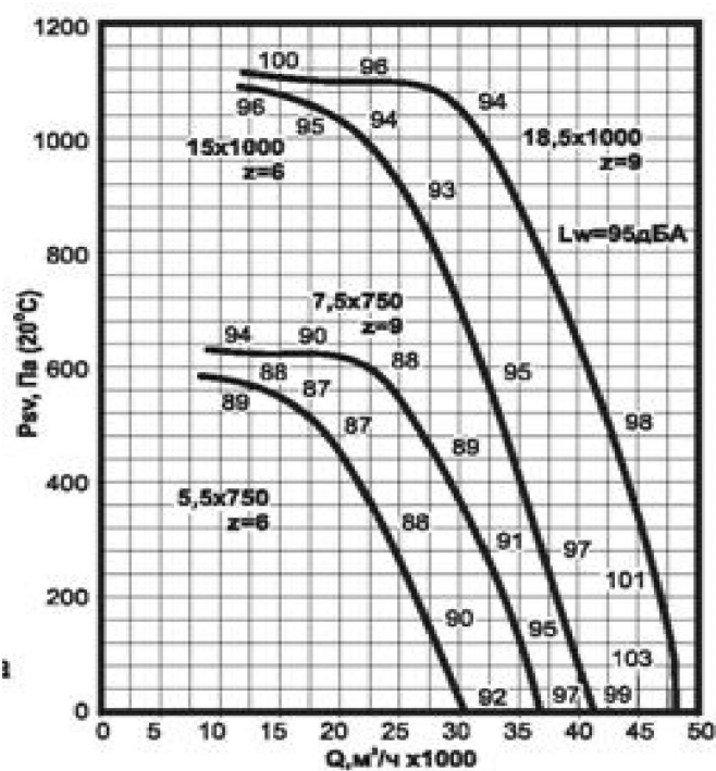
Аэродинамическая характеристика ВКРФ №10
