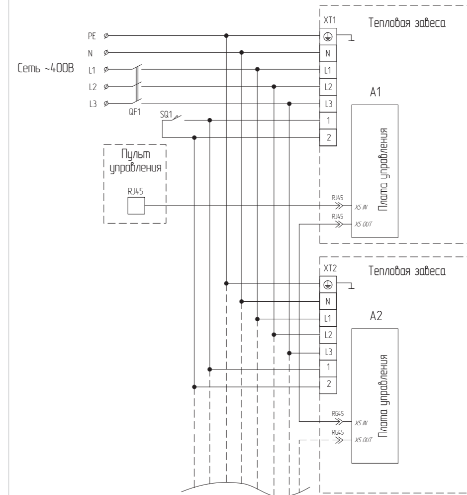
Групповое подключение завес с электрическим нагревом к пульту BRC-D1
