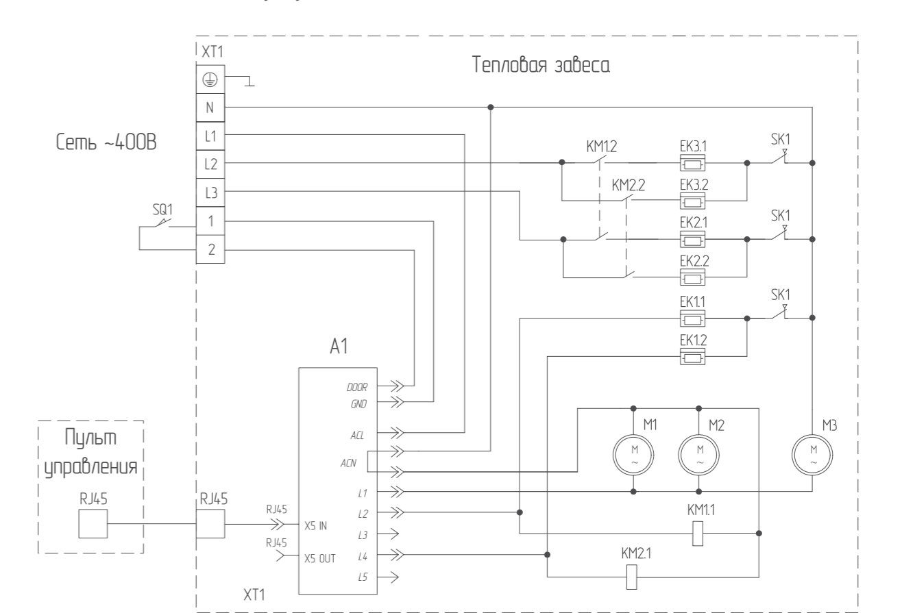
Подключение ВНС-L15-S09 (-М) к пульту ВНС-S
