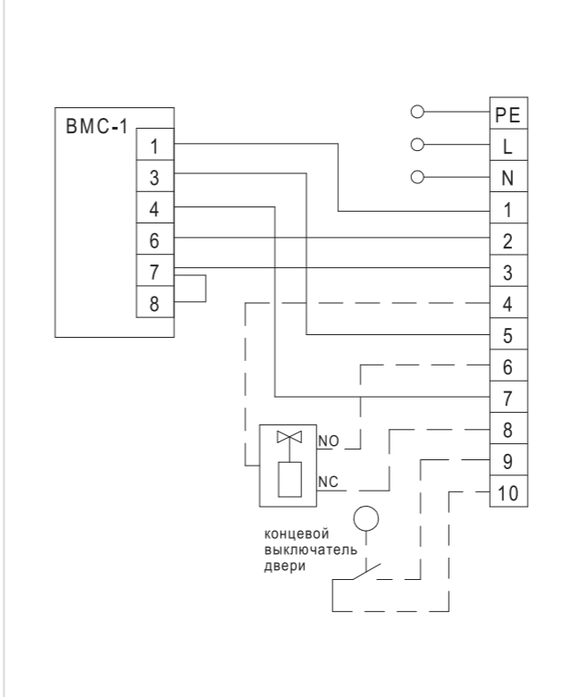
Подключение завес ВНС-Н15W30-SP, ВНС-Н20W45-SP к пульту ВМС-1
