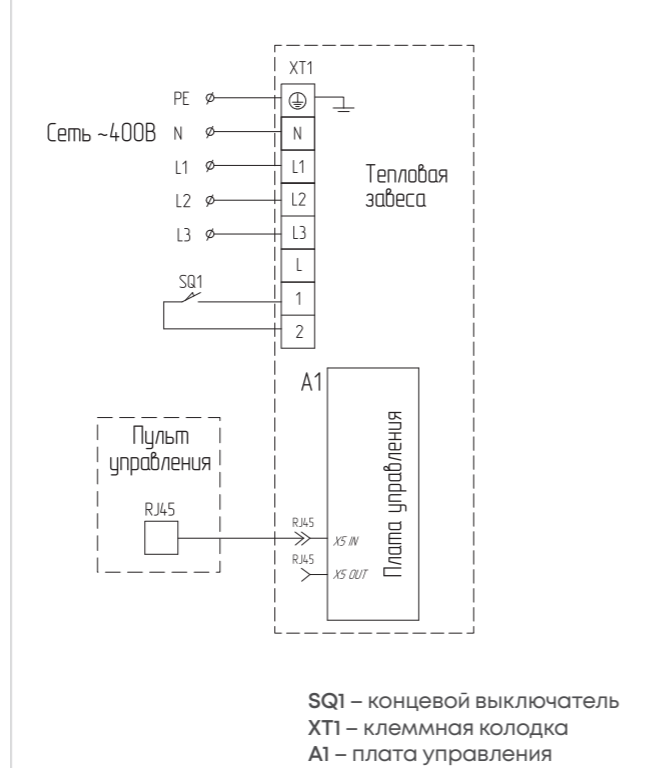
Подключение завес с электрическим нагревом к пульту BRC-D1
