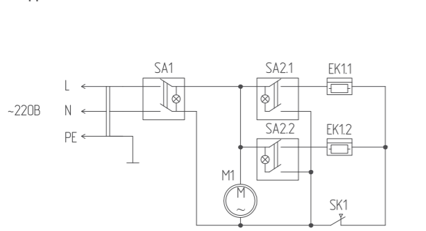
Подключение ВНС-L06-S03
