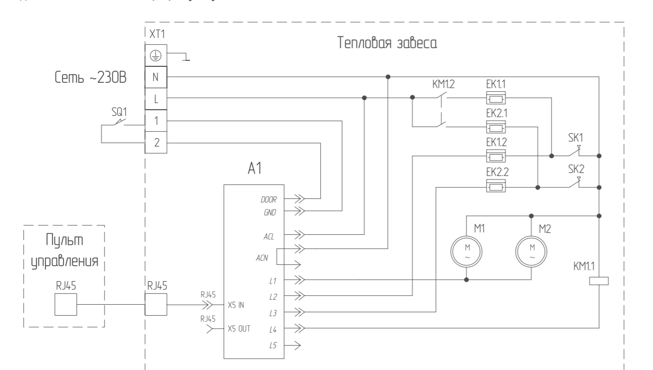
Подключение ВНС-L10-S06 (-М) к пульту ВНС-S
