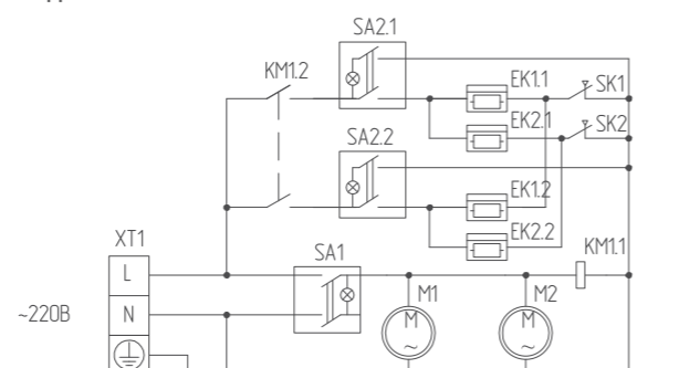
Подключение ВНС-L08-S05-M
