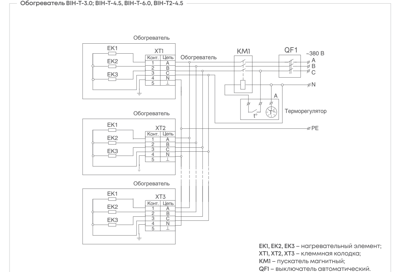
Обогреватель ВИН-T-3.0; ВИН-T-4.5, ВИН-T-6.0, ВИН-T2-4.5
