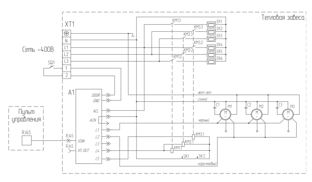
Подключение завес ULTRA с электрическим нагревом к пульту BRC-D1
