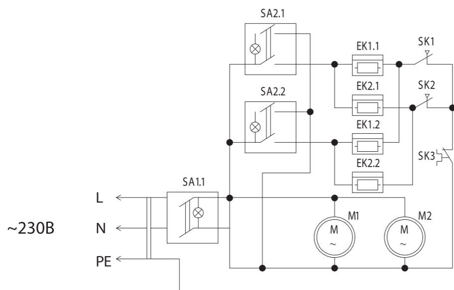
Подключение ВНС-СЕ-3Т
