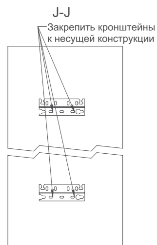
Схема крепления завес серии PS вертикально к стене с помощью кронштейнов
