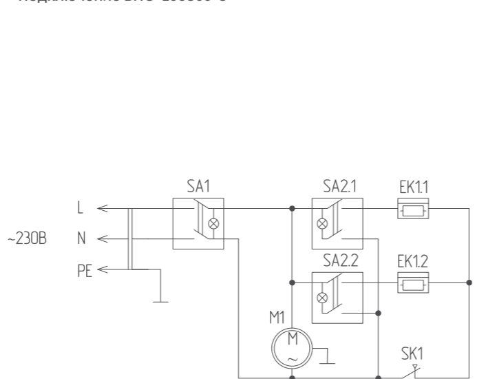
Подключение ВНС-L06S03-S
