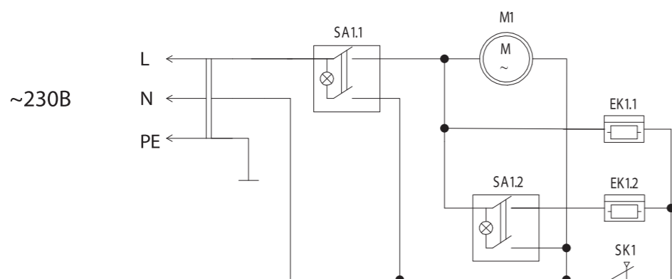
Подключение ВНС-СЕ-3 и ВНС-СЕ-3Л
