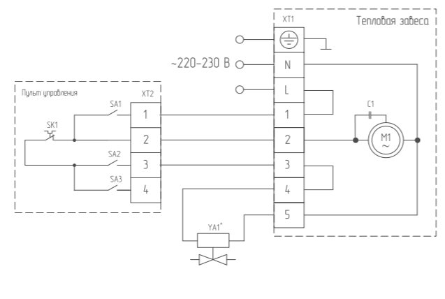
Подключение ВНС-В10W10-PS2 и ВНС-В15W15-PS2
