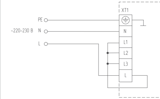
Подключение ВНС-В10Т06-PS2 к сети 230 В
