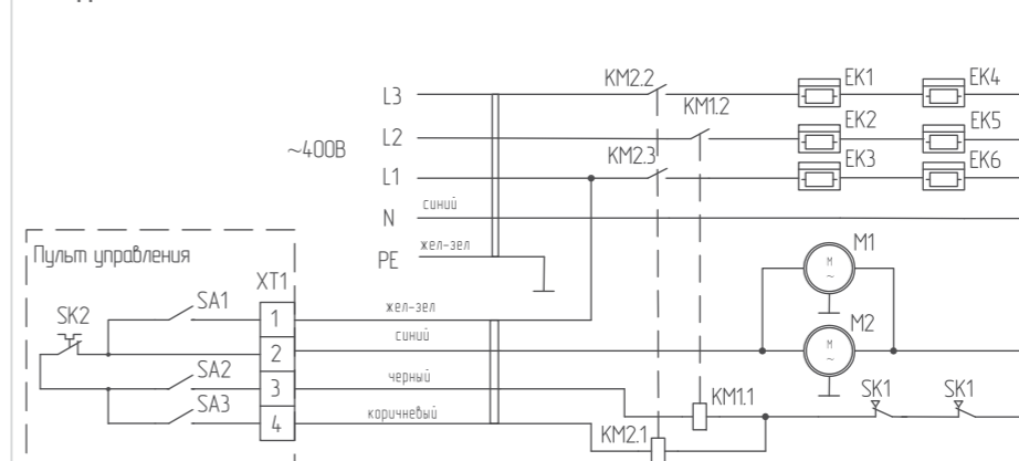
Подключение ВНС-L15S09-SP
