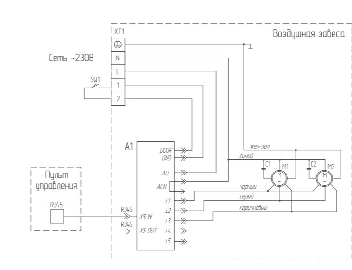
Подключение завес ULTRA без нагрева к пульту BRC-F
