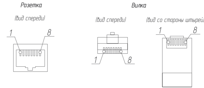
Схема обжимки проводов для подключения завесы к BMS
