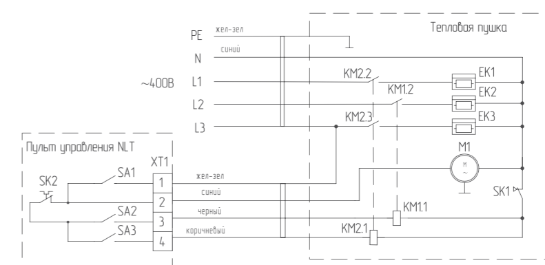
Подключение ВНР-MW-9 и ВНР-MW-15 к пульту NTL
