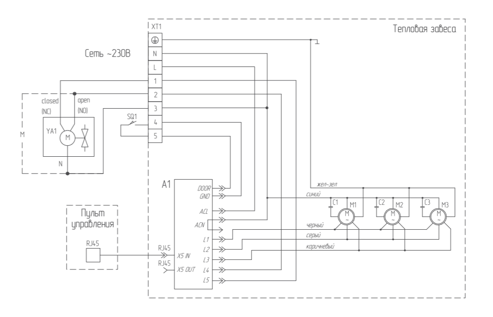
Подключение завес ULTRA с водяным теплообменником к пульту BRC-D2
