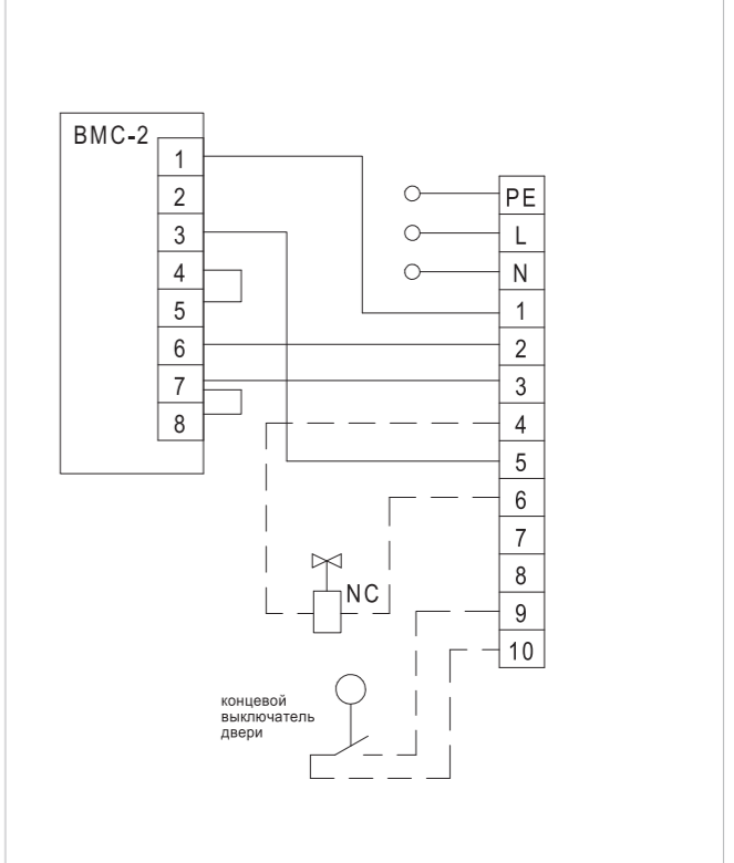
Подключение завес ВНС-Н15W30-SP, ВНС-Н20W45-SP к пульту ВМС-2
