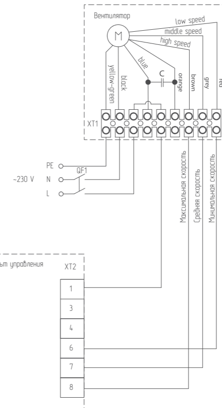
Подключение BDS-2-S к пульту BMC-1
