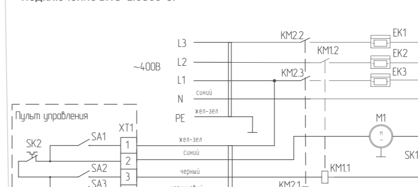
Подключение ВНС-L10S06-SP
