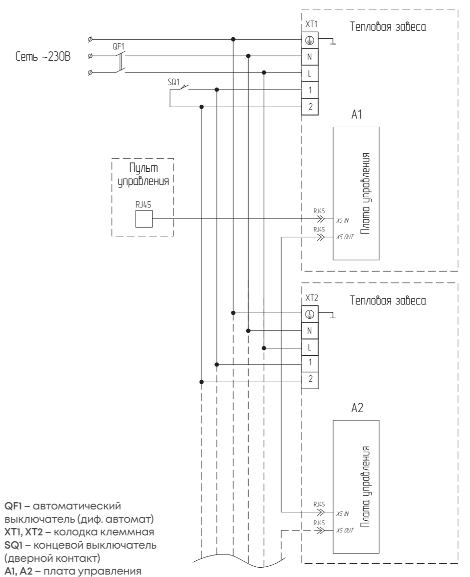
Групповое подключение завес без нагрева к пульту BRC-F
