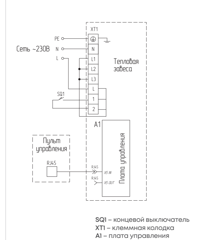
Подключение завес ВНС-М10Т06-PS (BRC-D1) к сети 230 В
