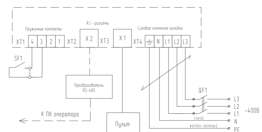
Подключение ВНР-MW2-10 и ВНР-MW2-15 к пульту BRC-D
