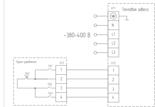
Подключение ВНС-В10Т06-PS2, ВНС-В15Т06-PS2, ВНС-В15Т09-PS2 и ВНС-В20Т12-PS2 к сети 400 В
