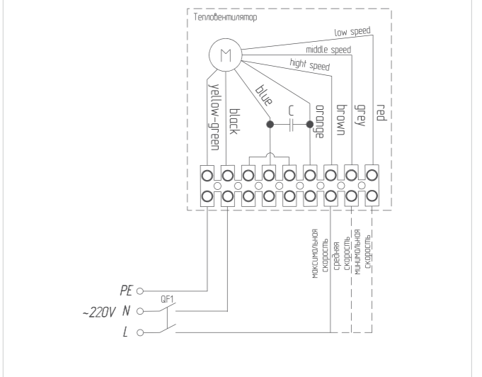
Подключение BDS-1-S к автоматическому выключателю
