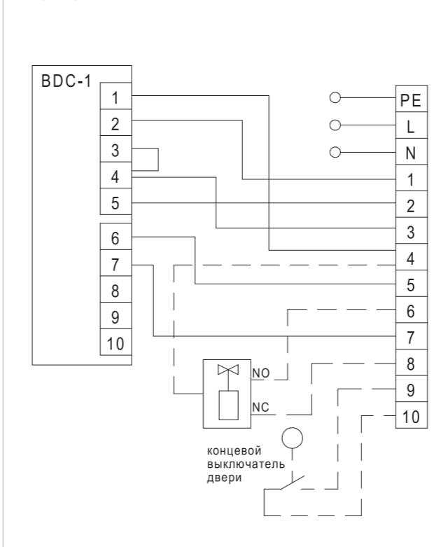
Подключение завес ВНС-Н15W30-SP, ВНС-Н20W45-SP к пульту ВДС-1
