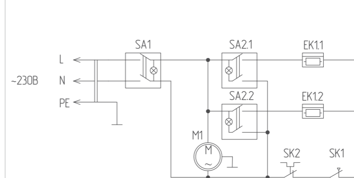
Подключение ВНС-L09S03-ST, ВНС-L09S05-ST
