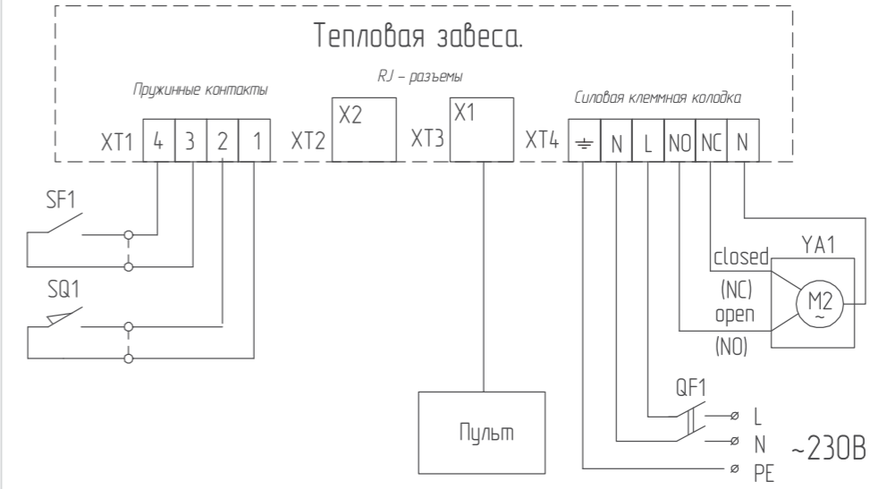
Подключение завес PS2 (Medium и High) с водяным теплообменником к пульту ВНС-D
