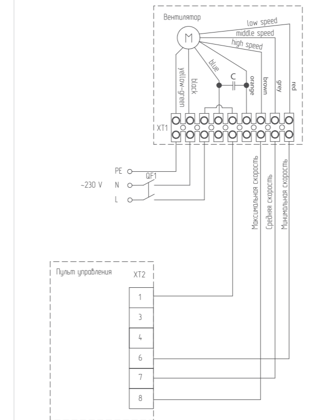
Подключение BDS-1-S к пульту ВМС-1
