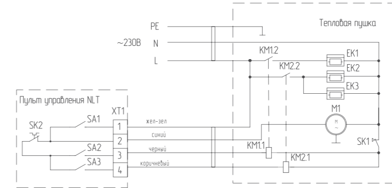
Подключение ВНР-MW-5 к пульту NTL
