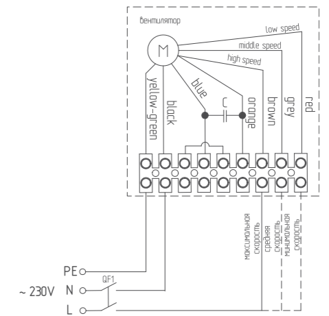
Подключение BDS-2-S к автоматическому выключателю
