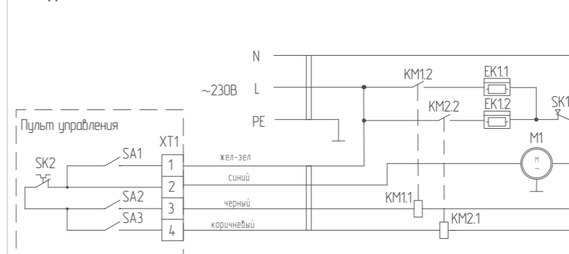
Подключение ВНС-L09S03-SP
