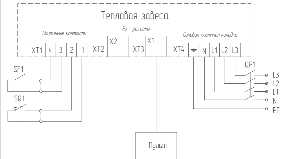
Подключение завес PS2 (Medium и High) с электрическим нагревом к пульту ВНС-D
