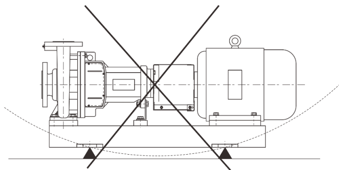
Рис. 8 Неправильный фундамент
