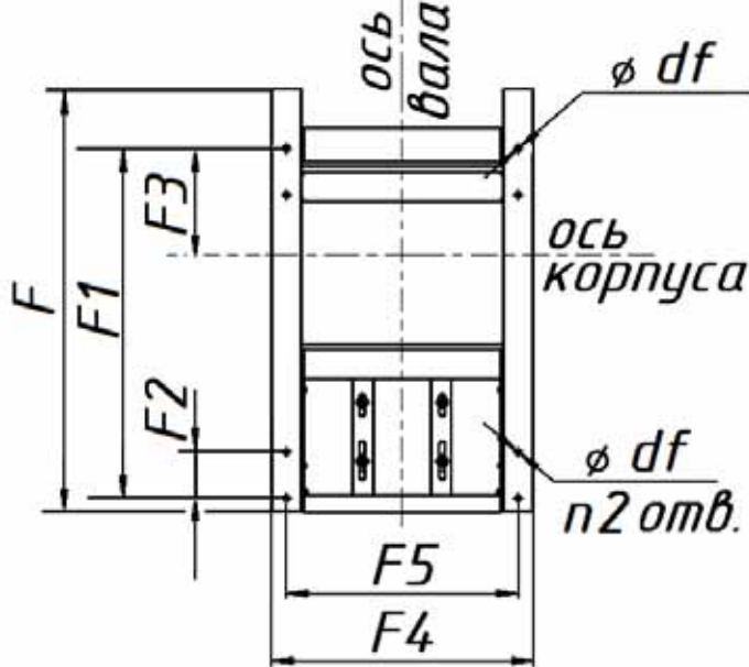
Основание монтажной рамы вид В
