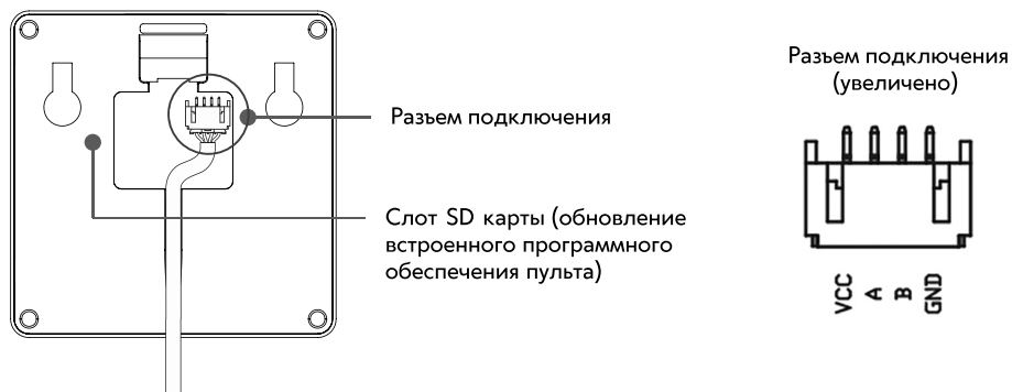
Рис. 8. Подключение к пульту управления
