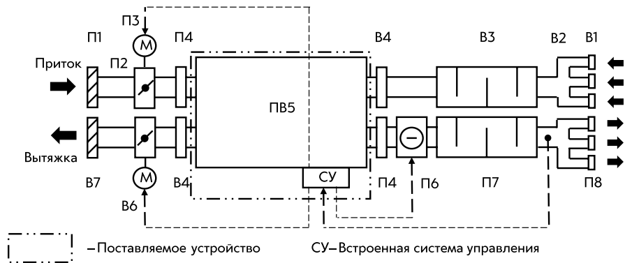
Рис. 6. Рекомендуемая структура и состав системы вентиляции
