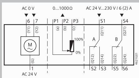
3-точечный, 24 В пер. тока
