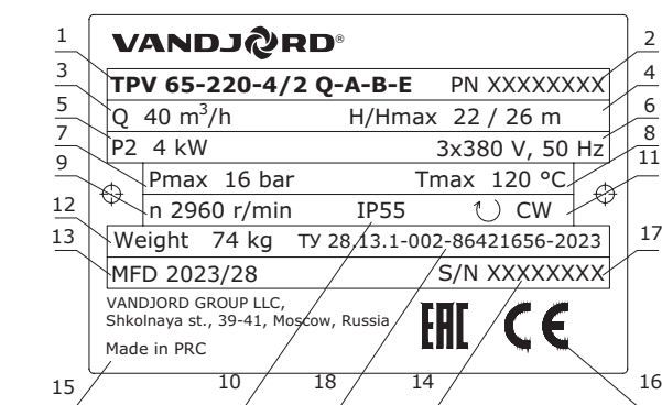
Рис. 3 Пример фирменной таблички насосов TPV
