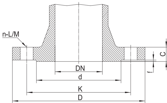
Рис. 18 Характеристики фланцев
