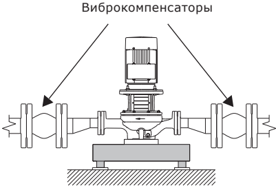
Рис. 11 Насос TPV с виброкомпенсаторами большего размера
