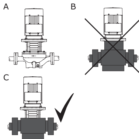
Рис. 12 Изоляция насосов TPV
