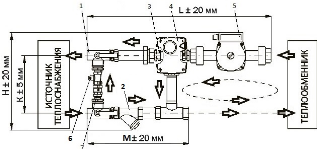
Схема смесительных узлов обратной конфигурации с байпасом
