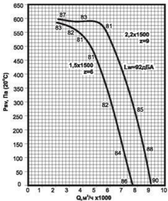
Аэродинамическая характеристика ВКРФ №5
