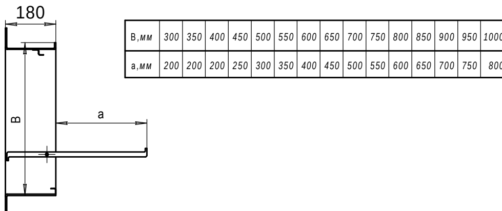
Рис. 2. Вылет заслонки за пределы корпуса клапана
