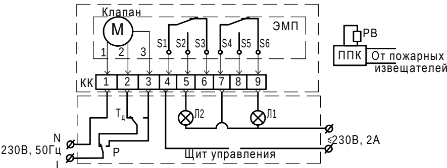
Рис. 8. Пример электрической схемы подключения клапана с реверсивным приводом без возвратной пружины типа 342..., 362... фирмы GRUNER или R-BLM фирмы Belimo.
