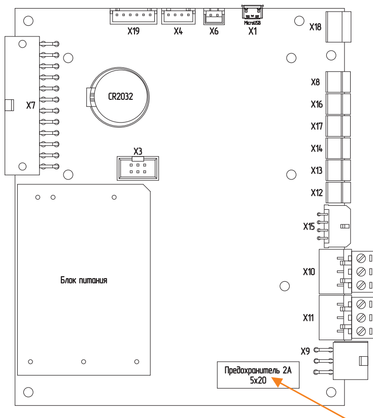
Рис.16 Плата контроллера
