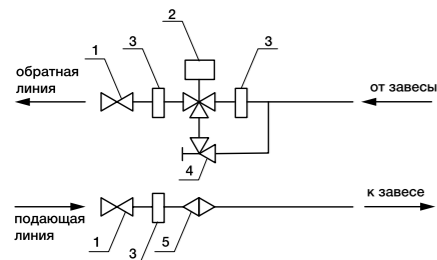
Схема 1 MST Eco Kv (Δp>40 кПа)
