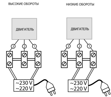
Схема 1 FLOW 100, 125
