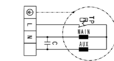
Схема 4
