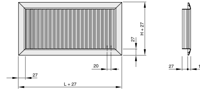
L Номинальная длина H Номинальная высота
