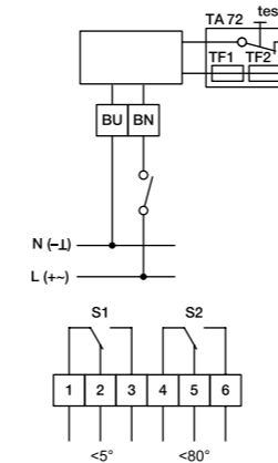
Схема 1 Серия 340
