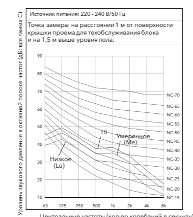
ESVMD-SF-90
