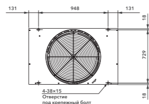
ESVMO-SF-335-A/400-A/450-A
