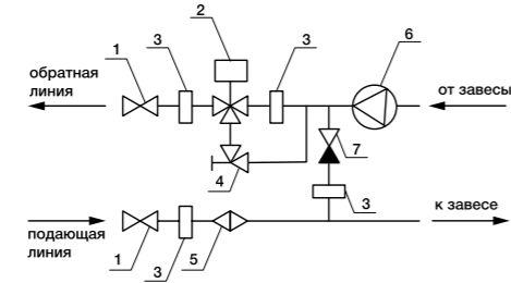
Схема 1 MST H Kv (Δp<40 кПа)
