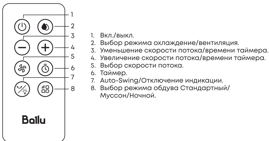
Рис. 3. Пульт ДУ.
