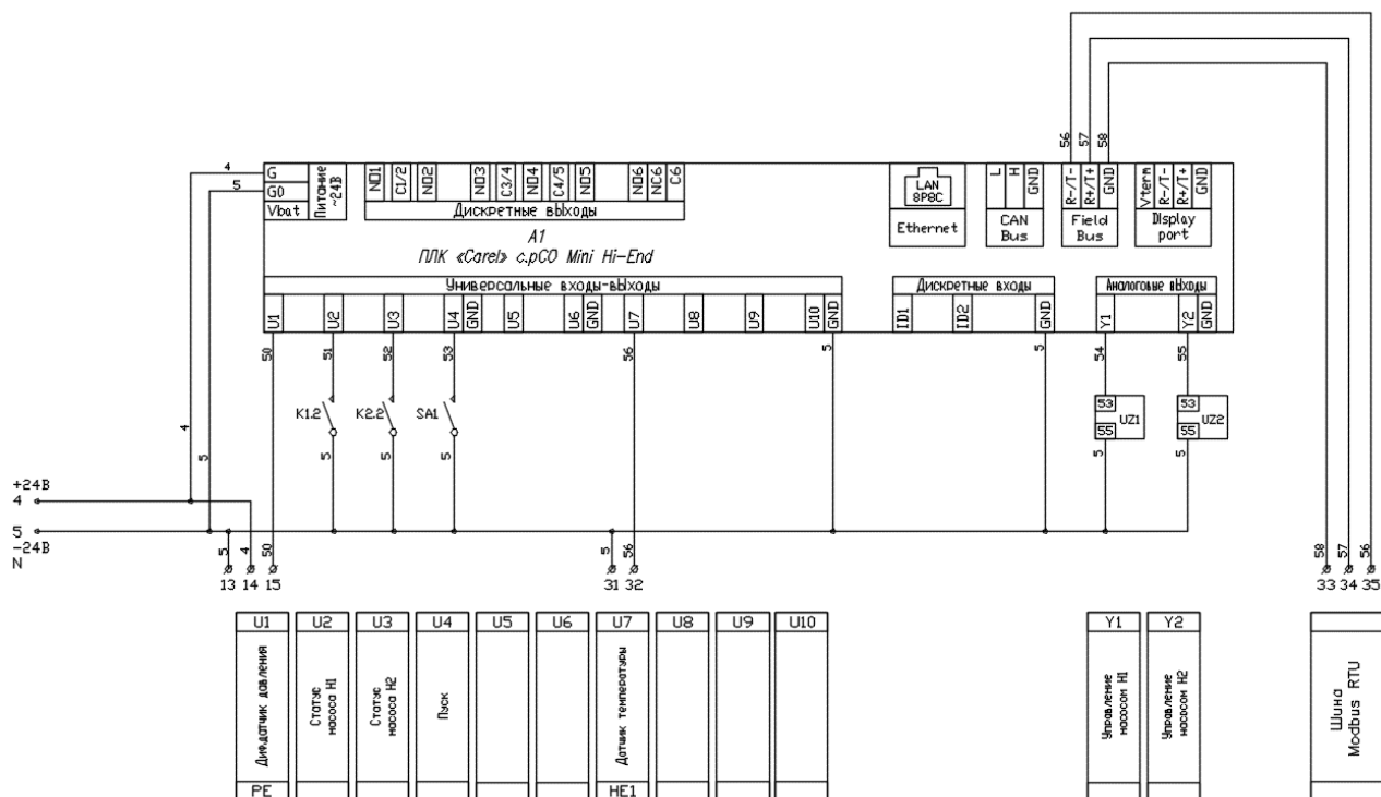
Рис. П1.2. Принципиальная электрическая схема шкафа электроподключений гидромодуля во внутреннем исполнении.
