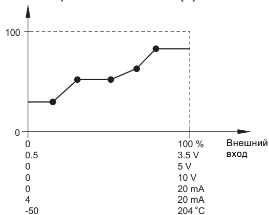
Рис. 78 "Таблица регулирования", пример с пятью точками
