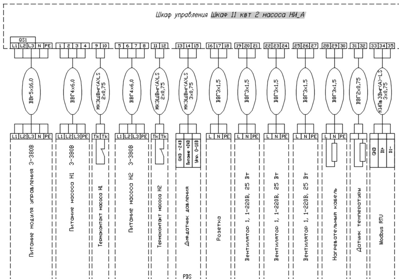
Рис. П1.3. Схема внешних подключений гидромодуля без системы автоматизации во внутреннем исполнении.
