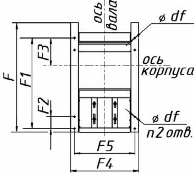
Основание монтажной рамы вид В
