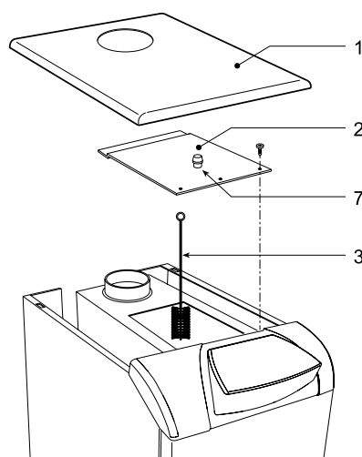
рис. 21 - Очистка котла
