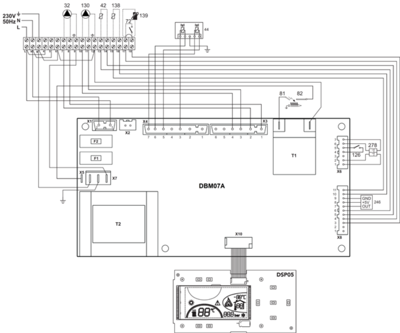
рис. 26 - Электрическая схема А
