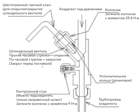
Размер шестигранного ключа (мм)
