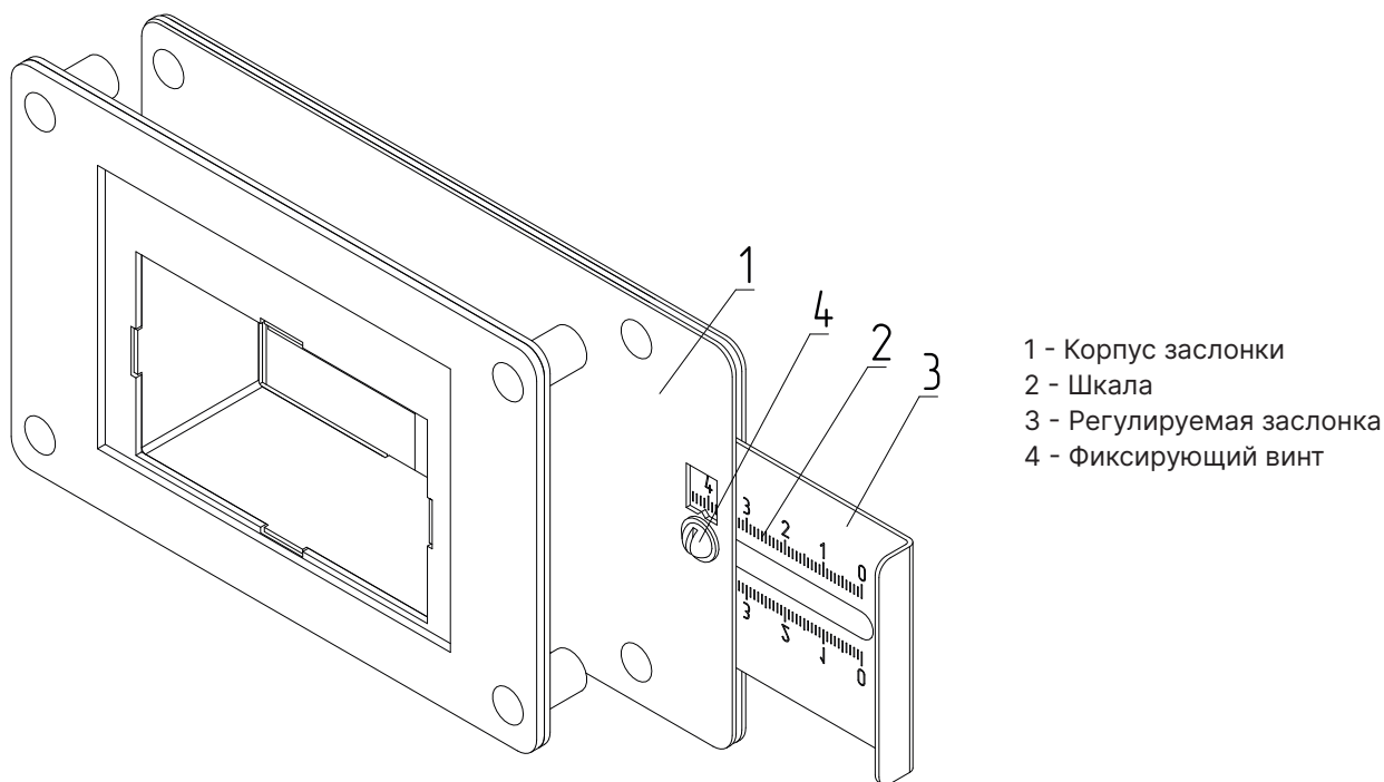
Рис.16 Заслонка вентилятора
