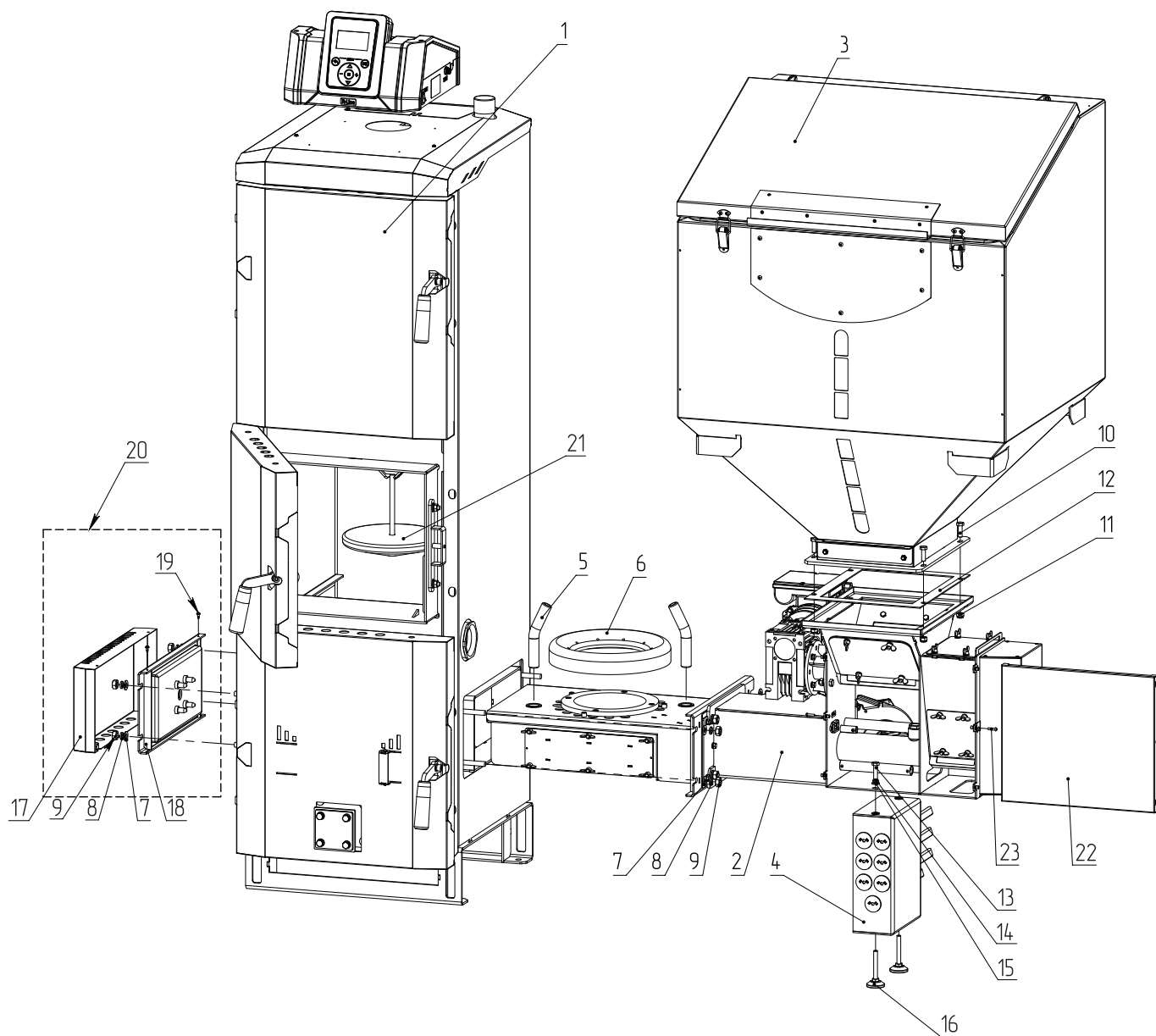
Рис.9 Монтаж котла
