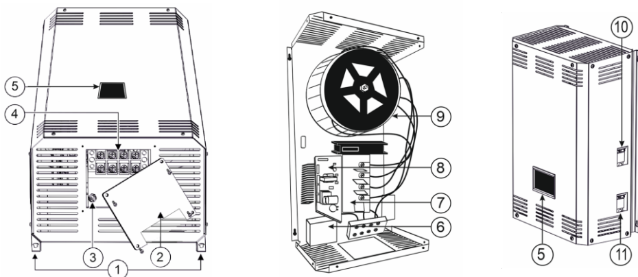
Рисунок 1 - Общий вид стабилизатора и его функциональных блоков
