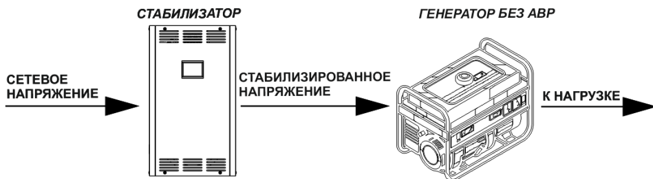
Рисунок 8 - Конфигурация 2 (размещение стабилизатора перед генератором)
