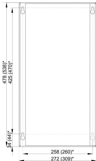
Рисунок 3 – Крепление изделия на стену (размеры со звёздочкой* — для ST-20000 LED, ST-30000 LED )
