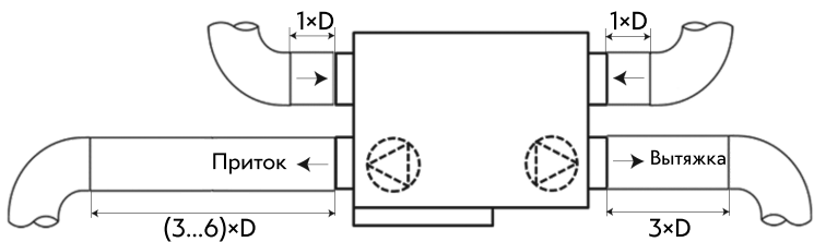
Рис. 13. Рекомендации по длине прямых участков воздуховода
