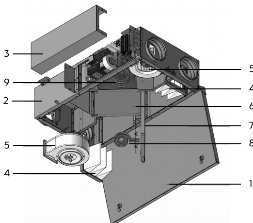
Рис. 1. Состав установки UniMAX-P 450 CE-A
