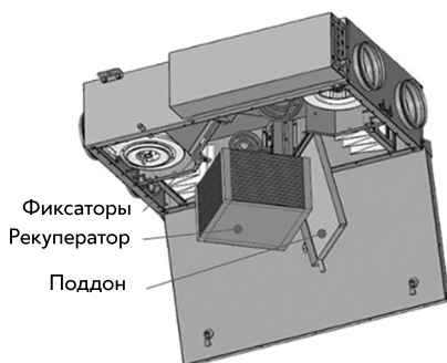
Рис. 38. Обслуживание рекуператора на UniMAX-P 450/800 CE-A
