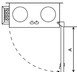
Рис. 10. UniMAX-P 450/800/1000 CE-A
