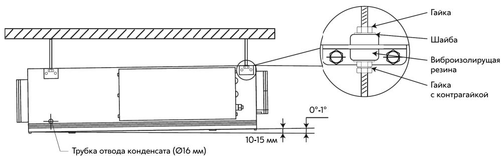
Рис. 9. Монтаж, дренажный уклон
