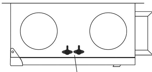
Рис. 24. Расположение портов для подключения трубок отбора давления
