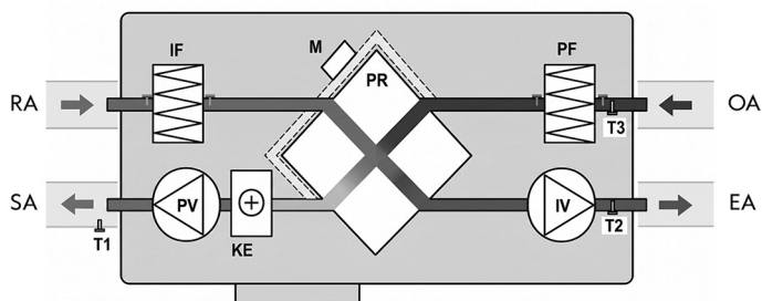
Рис. 6. Принципиальная схема UniMAX-P 1000/1500 CE-A
