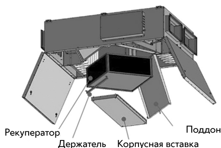
Рис. 40. Обслуживание рекуператора на UniMAX-P 1500 CE-A
