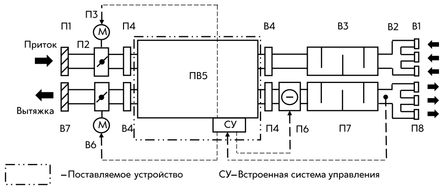
Рис. 7. Рекомендуемая структура и состав системы вентиляции
