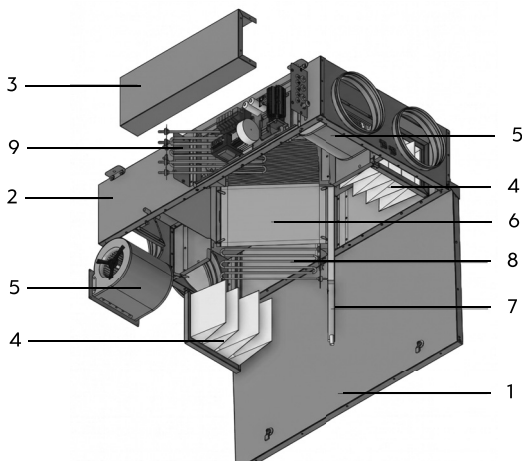
Рис. 2. Состав установки UniMAX-P 800 CE-A
