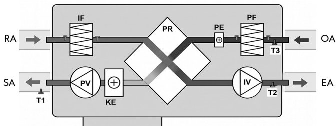
Рис. 5. Принципиальная схема UniMAX-P 450/800 CE-A
