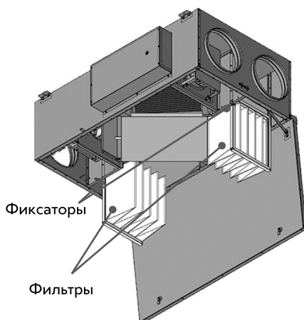
Рис. 37. Замена воздушных фильтров
