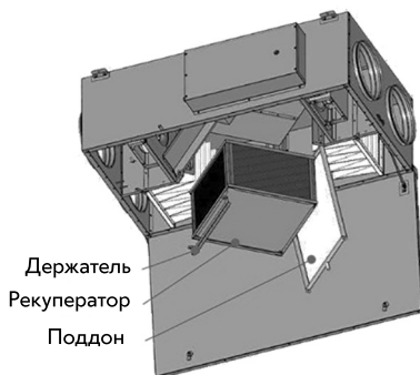
Рис. 39. Обслуживание рекуператора на UniMAX-P 1000 CE-A
