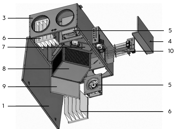
Рис. 3. Состав установки UniMAX-P 1000 CE-A
