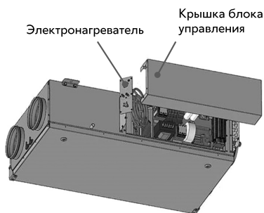
Рис. 42. Обслуживание электронагревателя
