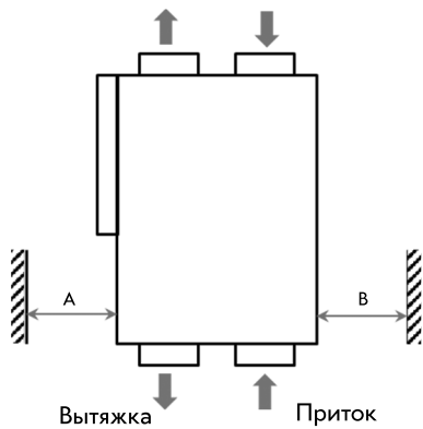
Рис. 12. Сервисное пространство
