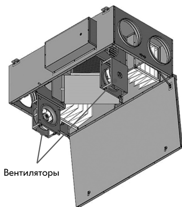
Рис. 41. Обслуживание вентилятора
