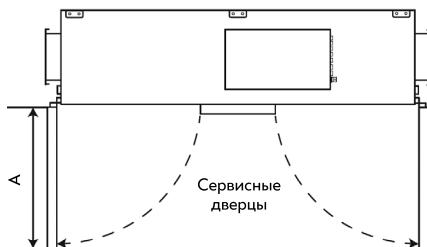
Рис. 11. UniMAX-P 1500 CE-A
