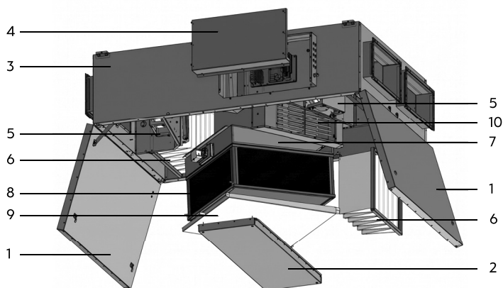
Рис. 4. Состав установки UniMAX-P 1500 CE-A
