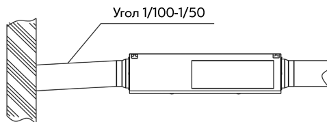
Рис. 15. Уклон наружных воздуховодов
