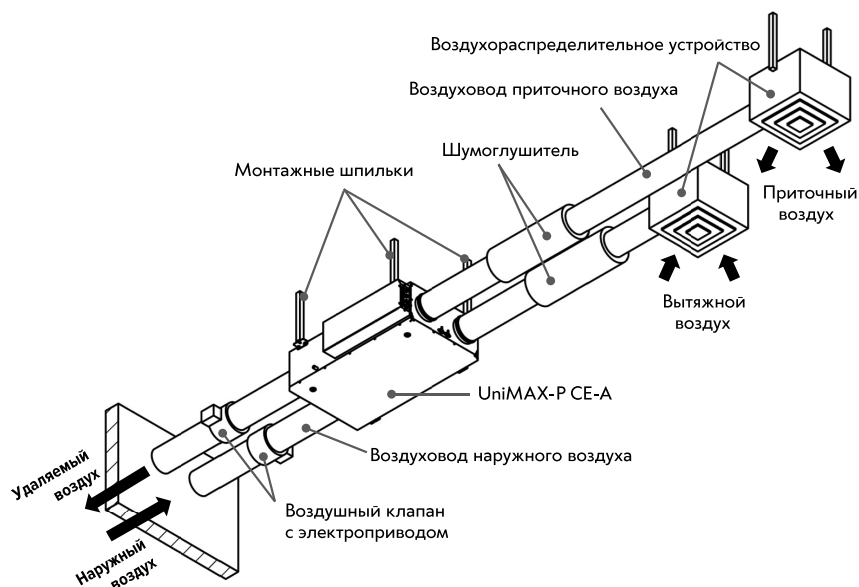
Рис. 17. Монтажная схема
