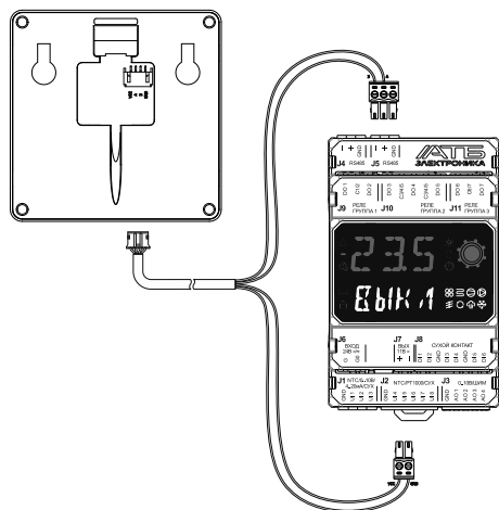
Рис. 21. Подключение к контроллеру
