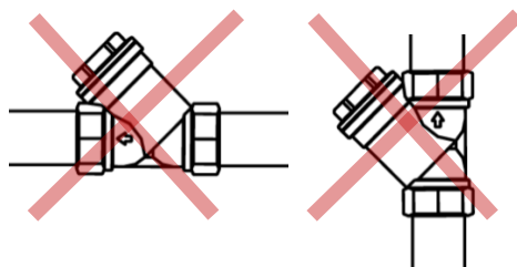
Рис. 7. Неправильный монтаж фильтра
