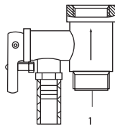
Рис. 1 Предохранительный клапан
