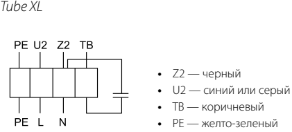
Схема электрических соединений
