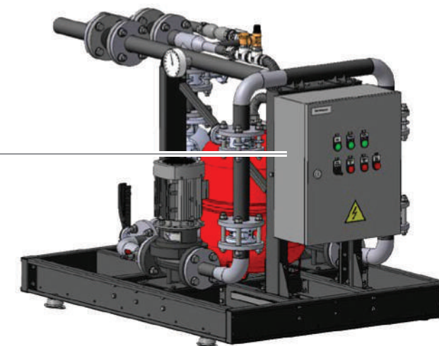
Шкаф электро- подключений
