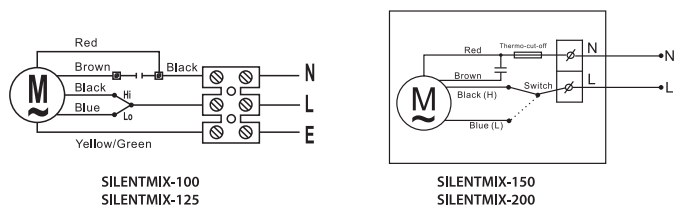
Рис. 3 Схема электрических соединений
