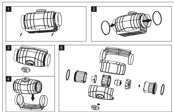
Рис. 2 Монтаж
