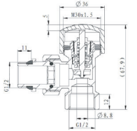
Угловой термостатический клапан
