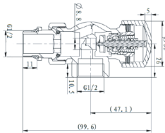
Осевой термостатический клапан
