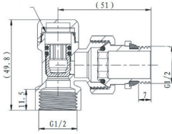
Угловой запорный клапан
