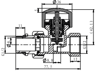
Прямой термостатический клапан
