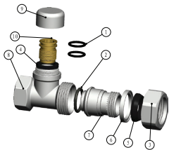
Прямой запорный клапан
