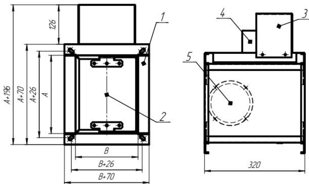
Рис. 1 Прямоугольный клапан с пределом огнестойкости EI 60.
