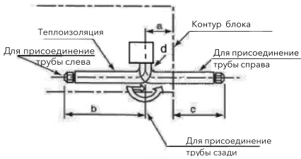
Жидкостная труба
