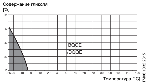
Рис. 5 Рабочий диапазон торцевых уплотнений из EPDM
