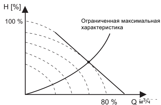
Рис. 64 Ограничения по мощности и давлению, влияющие на максимальную характеристику
