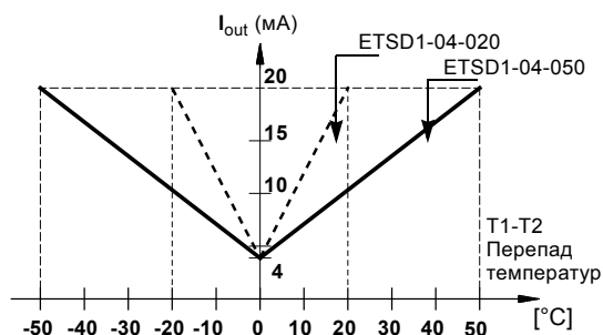
Рис. 118 Характеристики датчика
