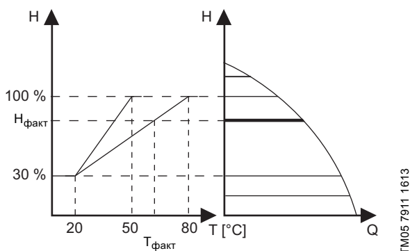
Рис. 82 "Влияние температуры"
