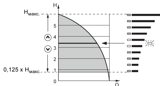
Рис. 39 Насос в режиме управления "Постоянного давления"
