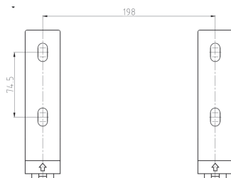
Рис. 8 Монтажные габариты комплекта настенного монтажа
