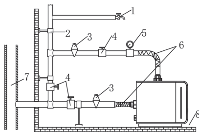
Рис. 11 Повышение давления воды из магистрального трубопровода
