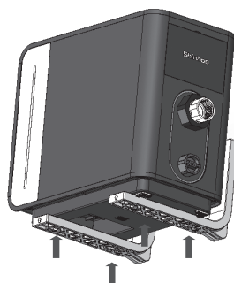
Рис. 9 Соединение комплекта настенного монтажа с установкой AQUAMASTER
