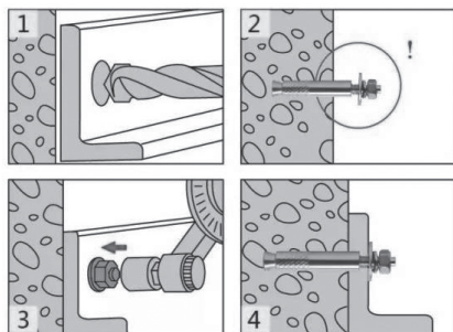
Рис. 5 Установка анкерных болтов
