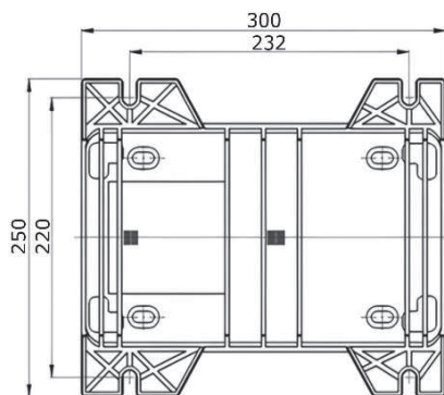
Рис. 21 Габаритный чертёж плиты-основания
