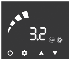
Рис. 15 Панель управления насосной установки AQUAMASTER
