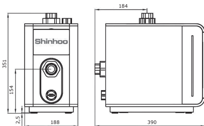
Рис. 20 Габаритный чертёж AQUAMASTER
