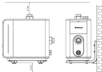
Рис. 7 Требуемое пространство при установке комплекта настенного монтажа
