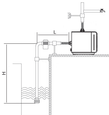
Рис. 13 Длина всасывающего трубопровода
