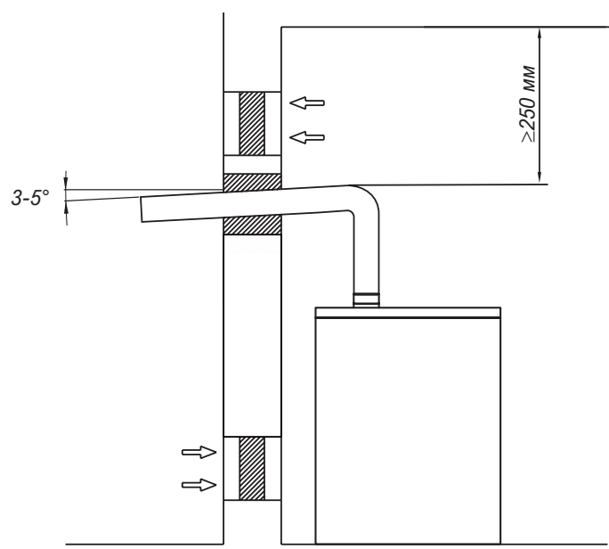
Рисунок 8. Система дымоудаления.
