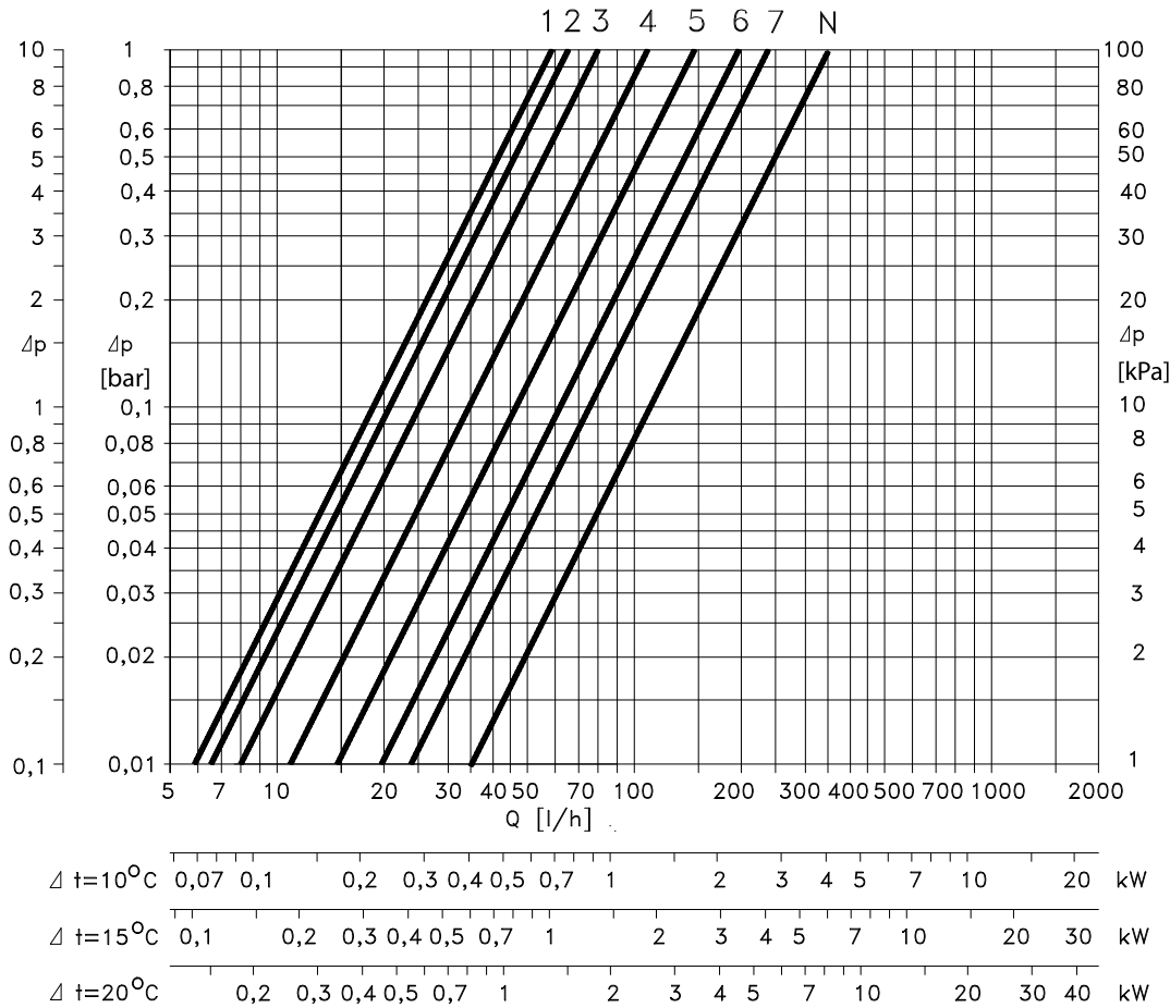
Диаграмма для определения предварительной настройки клапана RA-U 013G1383 с установленным термоэлементом серии RA 2000 при Хр=2°С
