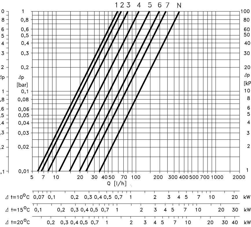
Диаграмма для определения пред- варительной настройки клапана RA-U 013G1383 с установленным термоз- элементом серии RA 2000 при Хр=2°C
