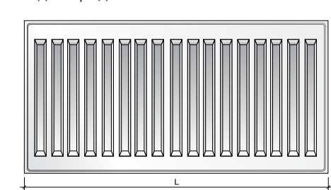
Вид спереди
