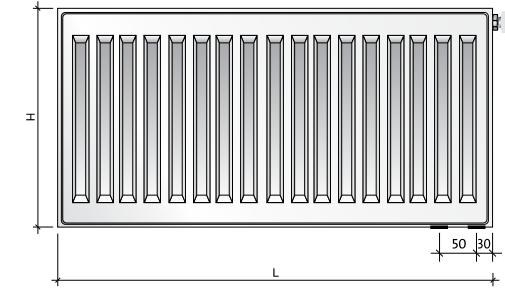
Вид спереди
