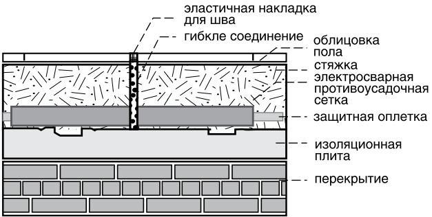
Рисунок 43. Схема укладки деформационного шва.
