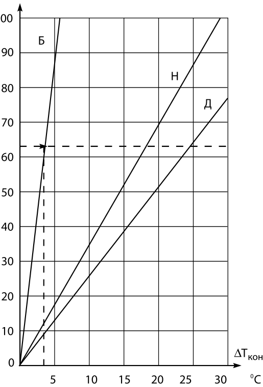
Рисунок 60. График понижения температуры в различных конструкциях пола.
